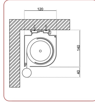
Tavan Montajı
