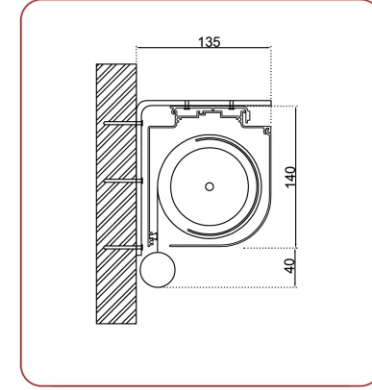
Duvar Montajı
